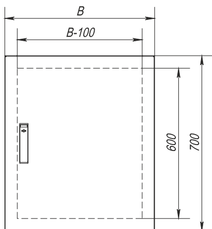
Вид спереди
