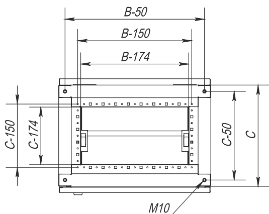
Вид сверху
