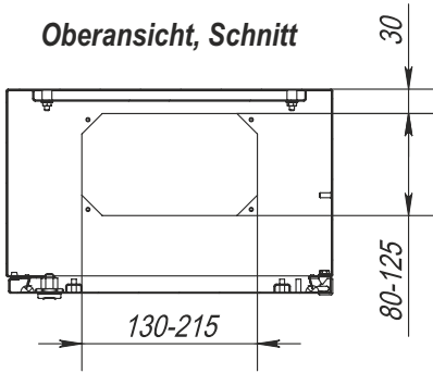
Montageplatte
