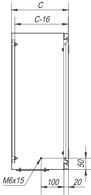
Linksansicht, Schnitt
