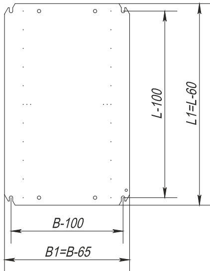
Montageplatte
