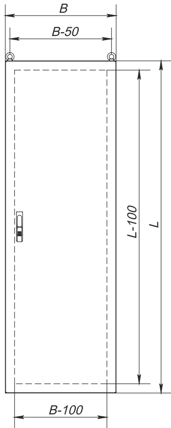
Frontansicht
