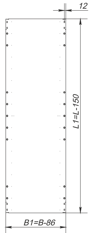
Montageplatte
