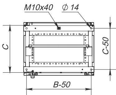
Oberansicht, Schnitt
