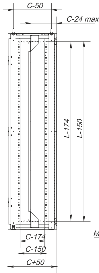
Linksansicht, Schnitt
