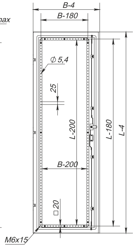
Tür, Innenansicht
