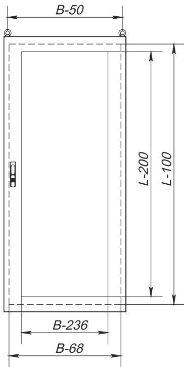
Frontansicht
