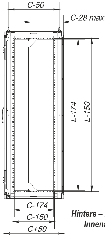
Linksansicht, Schnitt
