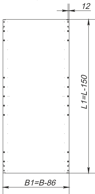
Montageplatte
