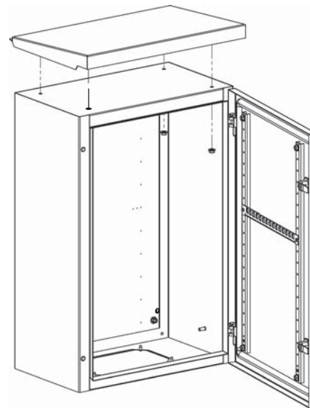
Установка дождевой крыши L-DK
