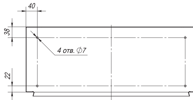
Разметка для установки дождевой крыши L-DK
