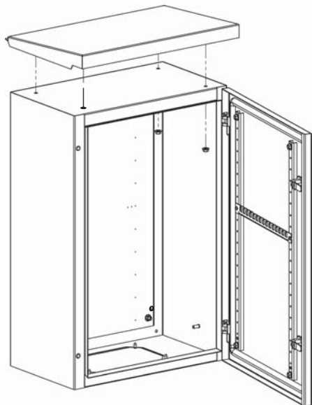
Установка дождевой крыши L-DK
