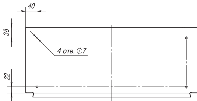
Разметка для установки дождевой крыши L-DK
