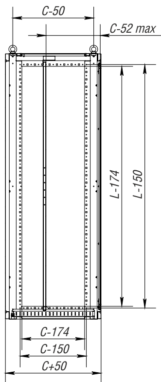
Вид слева, разрез
