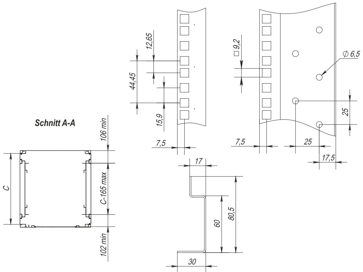
Montageprofil
